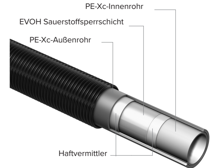
Aufbau des TECEflex PE-Xc 5S Rohres
