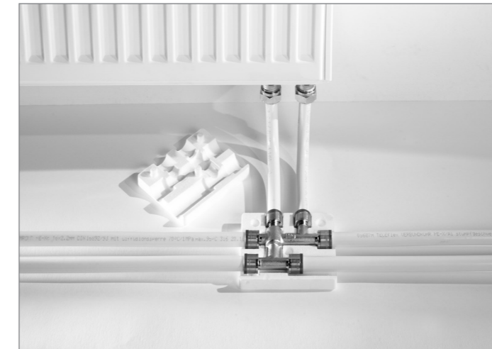
Heizkörperanschluss mit Kreuzungsfitting
